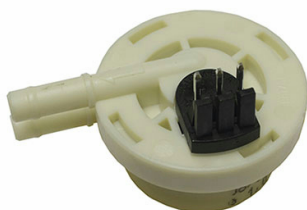
10070767 CONTATORE VOLUMETRICO
