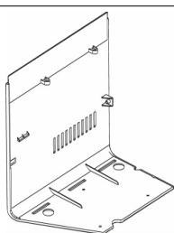
10070725 FIANCATA SX
