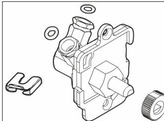
10070770 RUBINETTO VAPORE ASSEMBLATO
