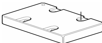
10085228 SOVRAPIASTRA X LABIRINTO INOX
