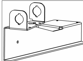
10079788 STAFFA DISTRIBUTORE
