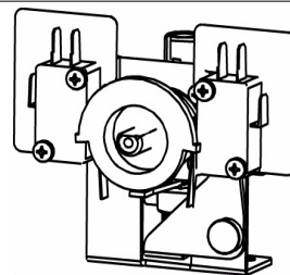
10079786 DISTRIBUTORE ASSEMBLATO
